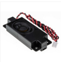
RS PRO 8Ω 2W Miniature Speaker, 40mm Lead Length, 80 x 31.1 x 14.9mm, Громкоговоритель (динамик)
